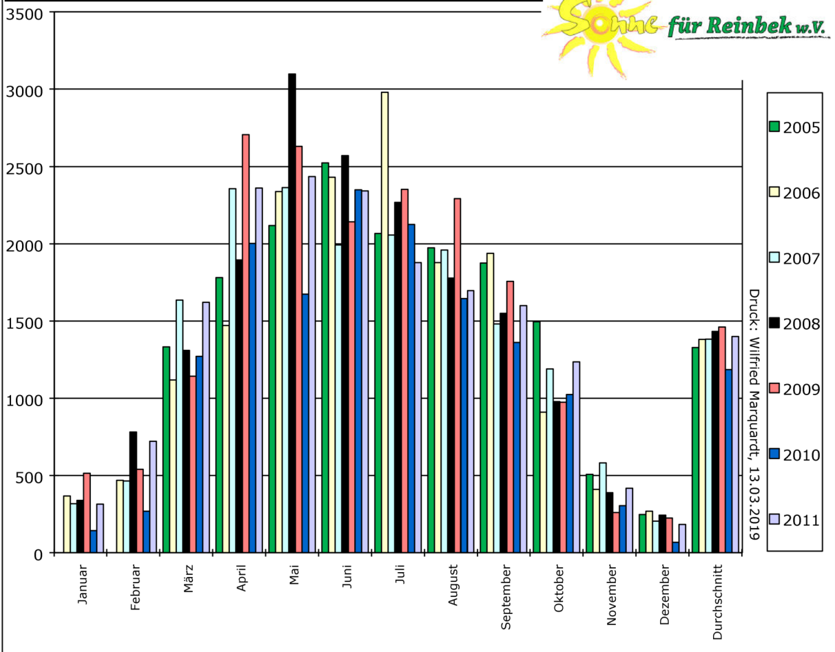
Erträge in Kwh: Gertrud-Lege-Schule von 2005 bis 2011
