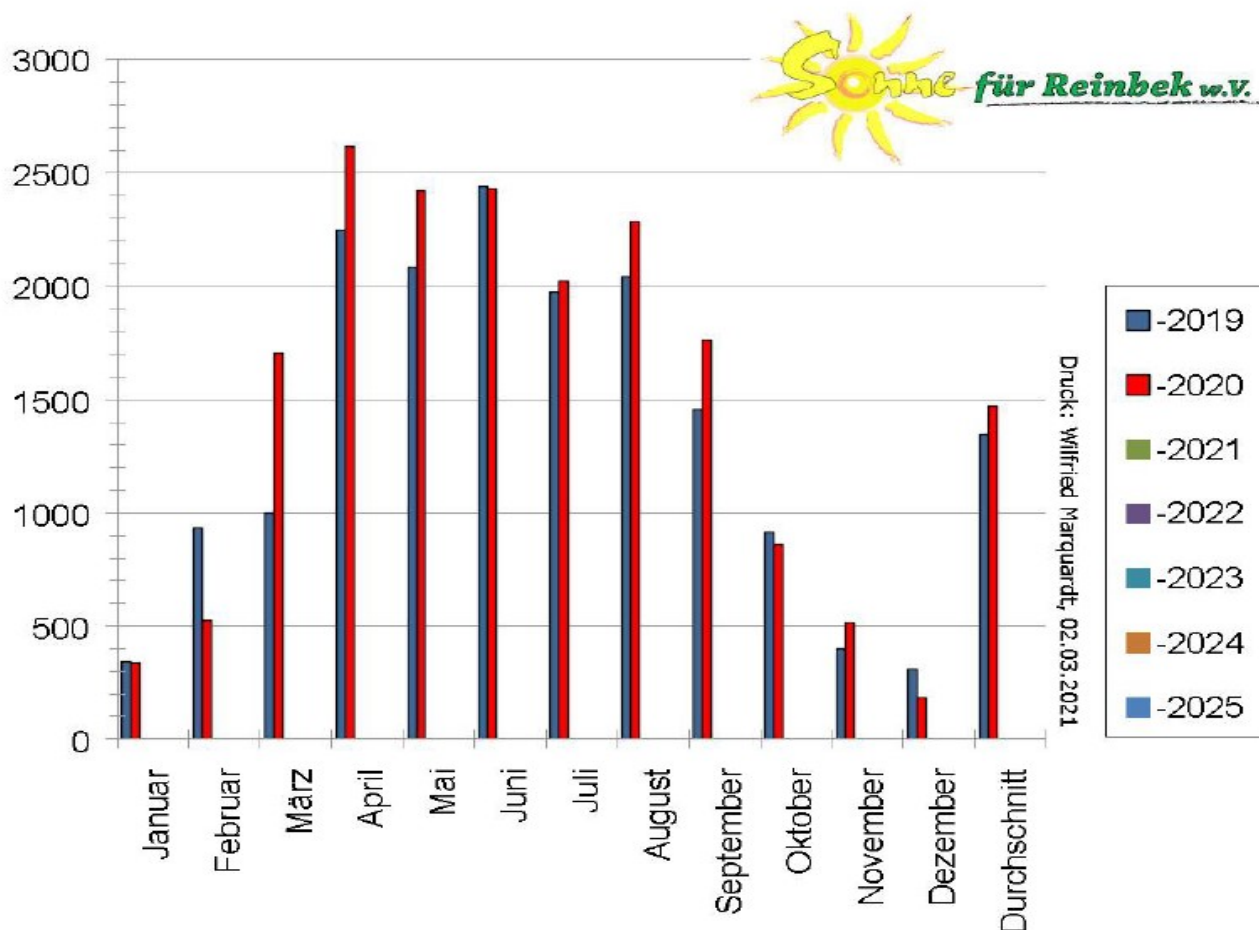
Diagramm 3: Gertrud-Lege-Schule, Erträge in Kwh 2019 bis 2025
